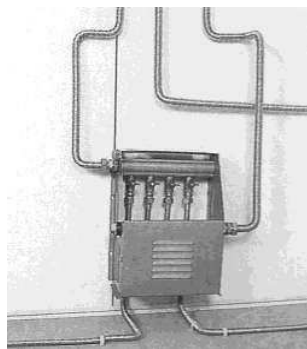
ที่ยึดหัวแบบตอก
